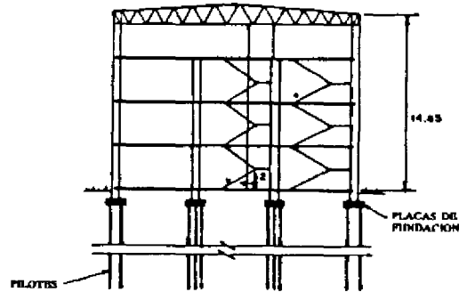
SECCION NORTE-SUR
