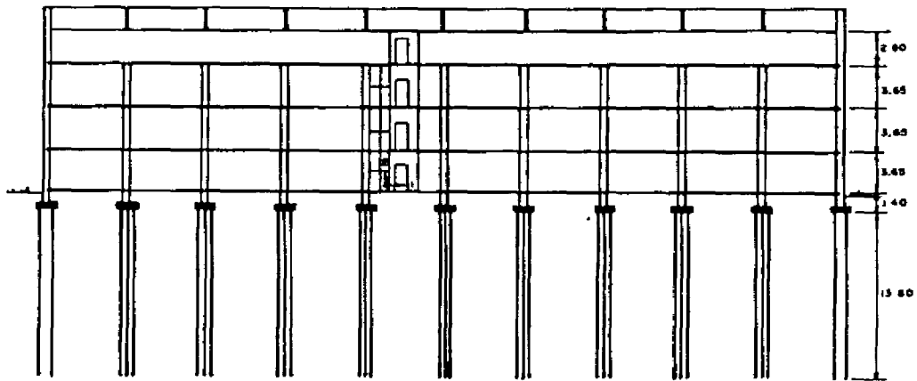
SECCION ESTE-OESTE
