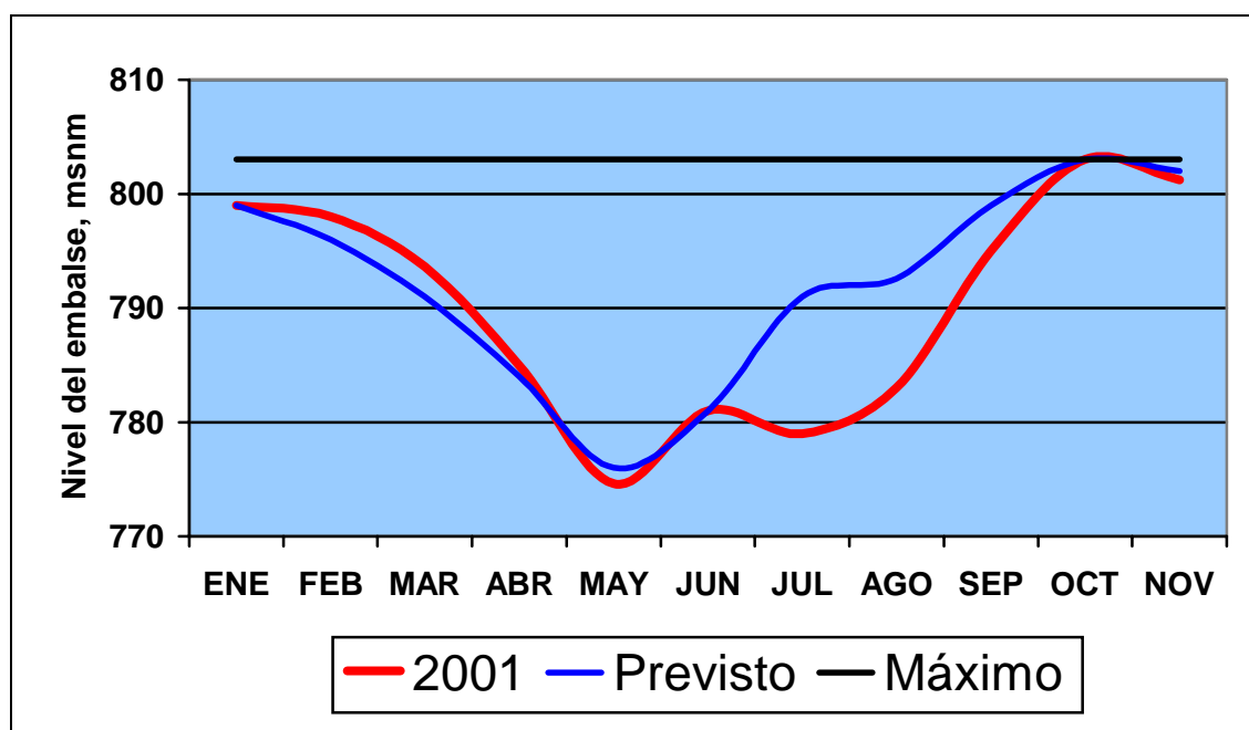
Gráfico 2-4. Variación del nivel del embalse de la central hidroeléctrica de Chixoy de Guatemala en 2001 En comparación con el nivel previsto y el nivel máximo permisible 33
