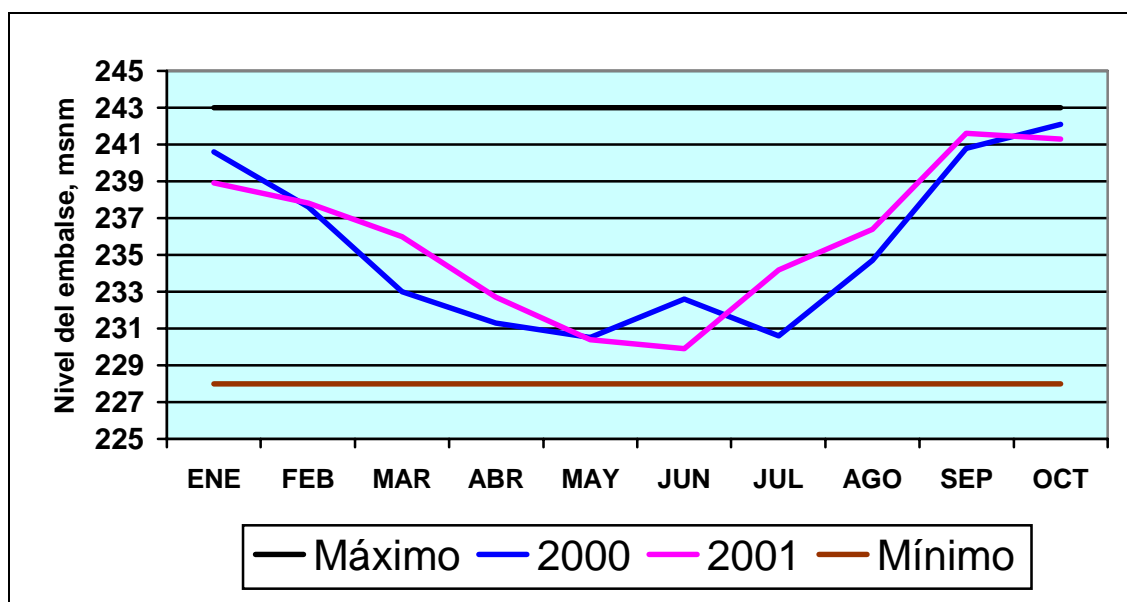
Gráfico 2-3. Variación del nivel del embalse de la central hidroeléctrica Cerrón Grande en El Salvador durante los años 2000 y 2001, en comparación con los niveles mínimo y máximo 32
