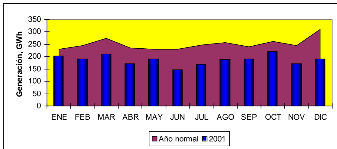
Gráfico 2-9. Generación de hidroelectricidad durante 2001 en Panamá en comparación con la de un año normal
