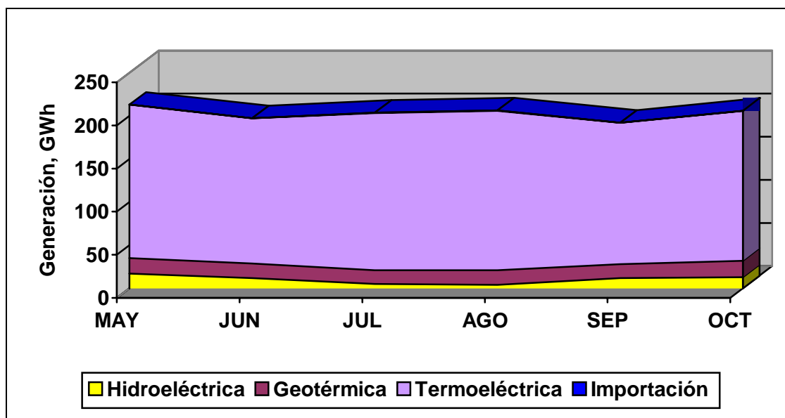
Gráfico 2-6. Generación eléctrica en Nicaragua durante la sequía de 2001 de acuerdo con el tipo de central 34
