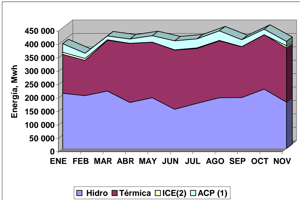
Gráfico 2-7. Generación eléctrica en Panamá durante la sequía de 2001, de acuerdo con el tipo de proveedor
