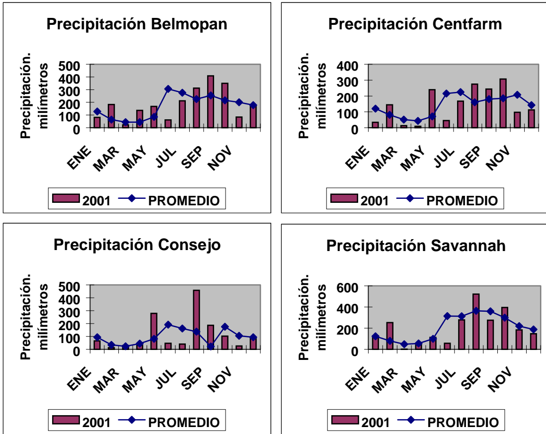
Gráfico 1-2. Precipitación mensual en 2001 y promedio de estaciones seleccionadas de Belice
