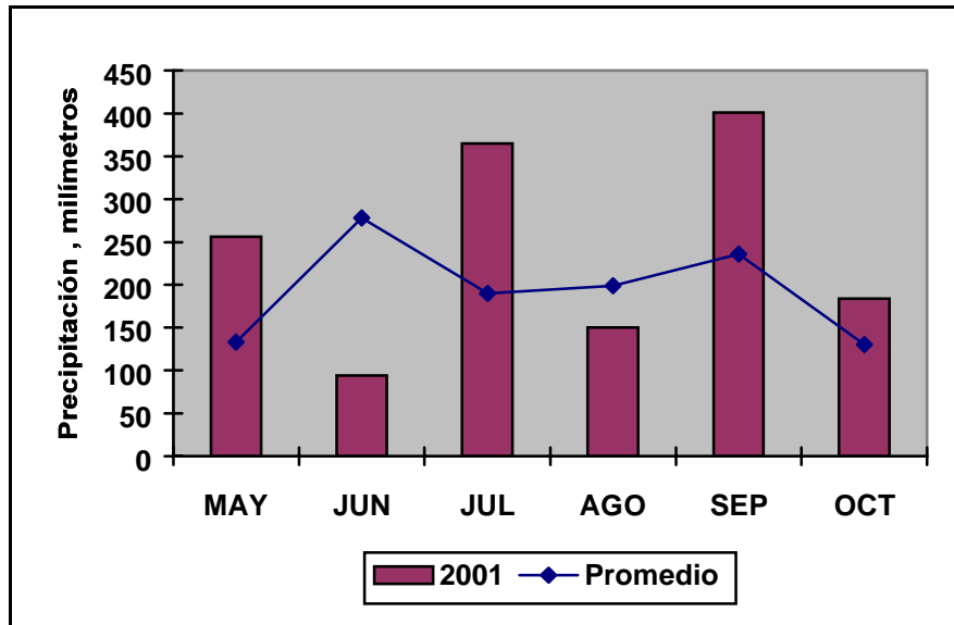
Gráfico 1-3. Precipitación mensual en 2001 y promedio histórico en la estación de Asunción Mita, Guatemala
