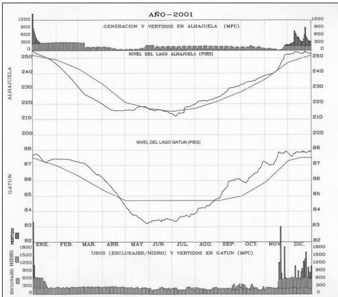
Gráfico 2-8. Generación hidroeléctrica, nivel y vertido de los embalses de la Cuenca del Canal de Panamá a/
