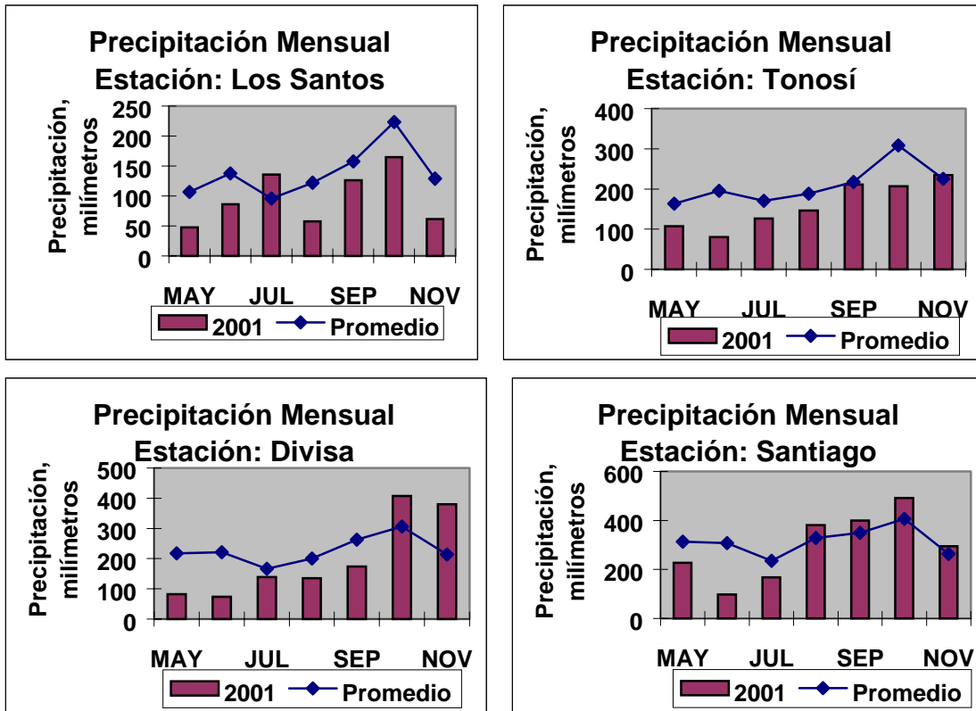
Gráfico 1-7. Precipitación mensual en 2001 y promedio histórico en estaciones de las provincias afectadas en Panamá
