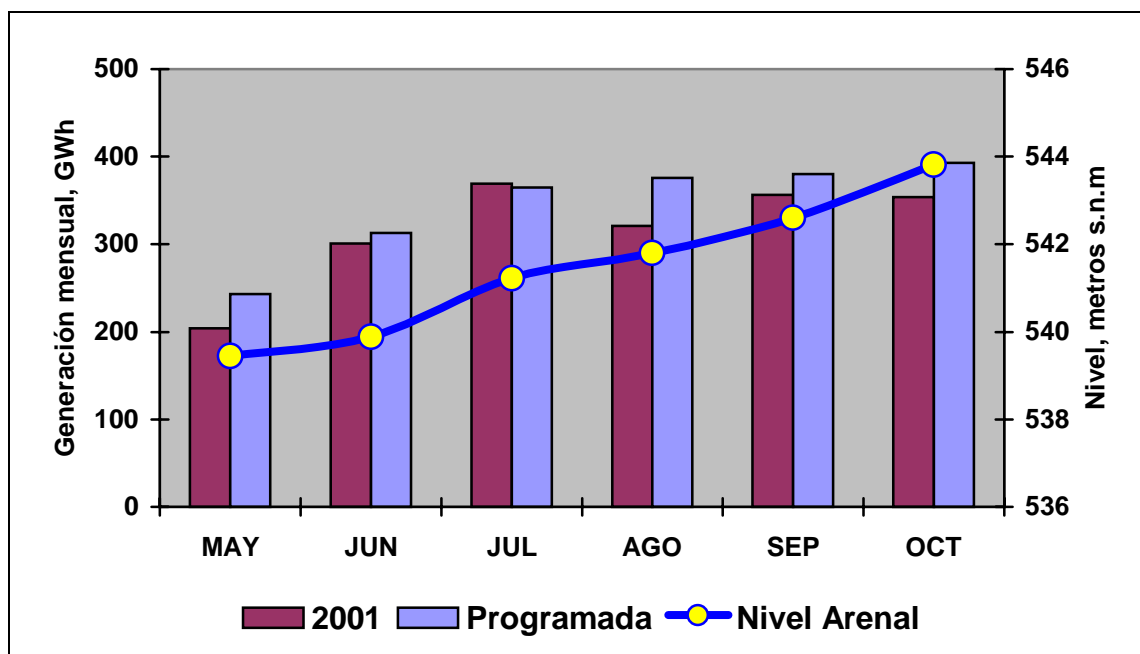
Gráfico 2-2. Comparación entre la generación programada y la efectuada en Costa Rica durante 2001 y la variación del nivel del embalse Arenal 31
