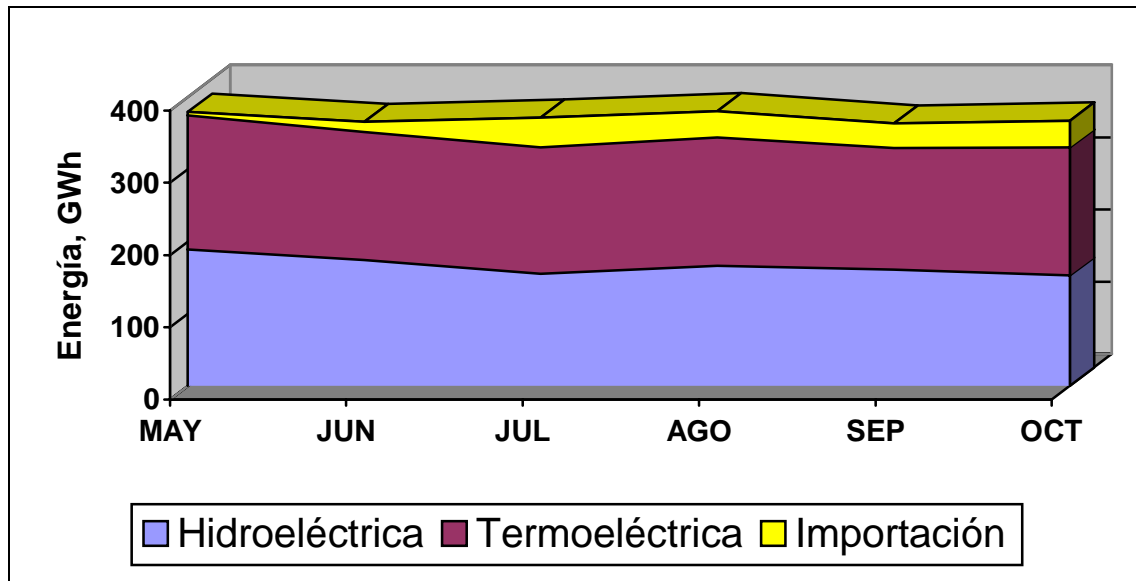
Gráfico 2-5. Distribución de la generación eléctrica en Honduras durante el período mayo a octubre de 2001
