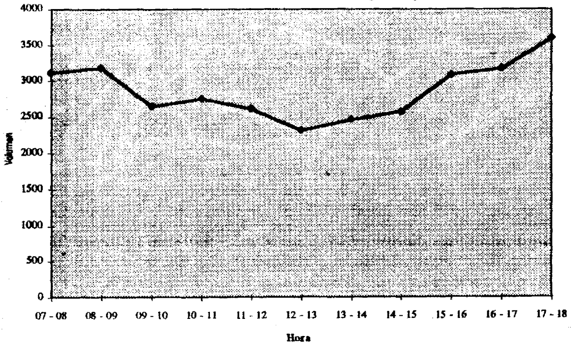
FIGURA 3 Perfil de Variación Horaria Ruta 1 (Antiguo Peaje)
