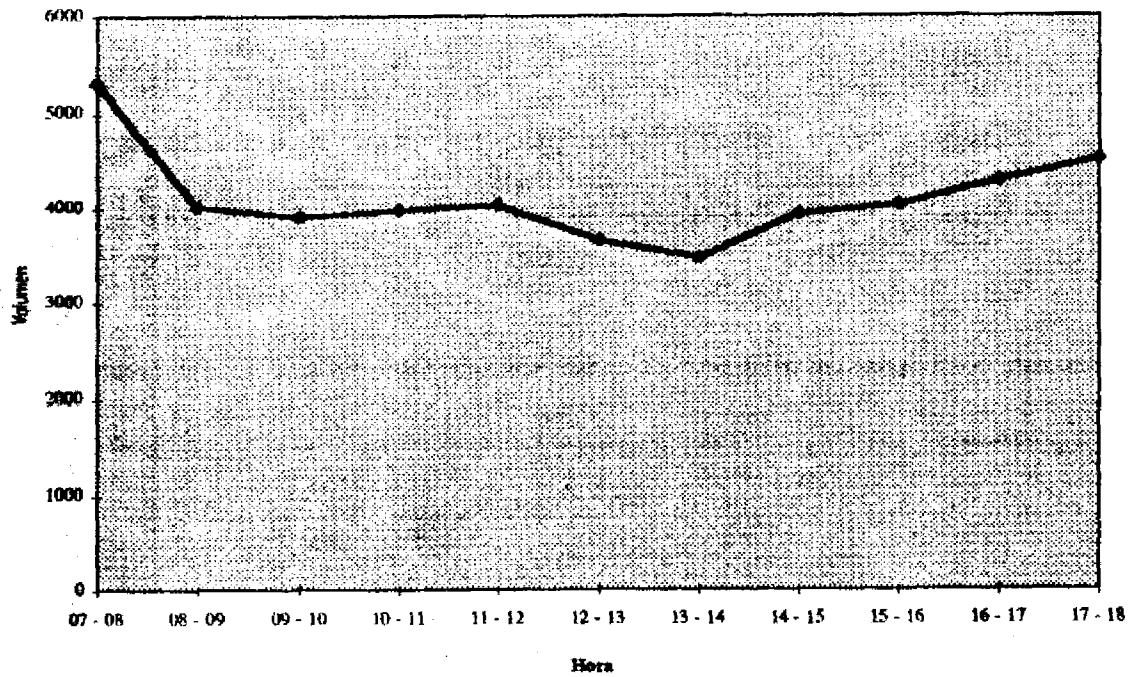
FIGURA 1 Perfil de Variación Horaria Ruta 1 (Río Torres)
