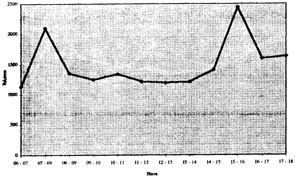
FIGURA 7 Perfil de Variación Horaria Ruta 2 (Tres Ríos)
