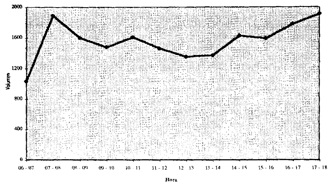
FIGURA 10 Perfil de Variación Horaria Ruta 3
